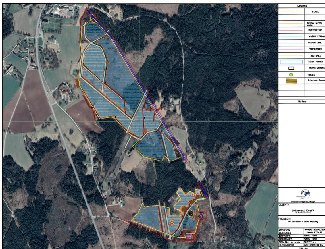
FIGUR 1. LAYOUT GÄLLSTAD
